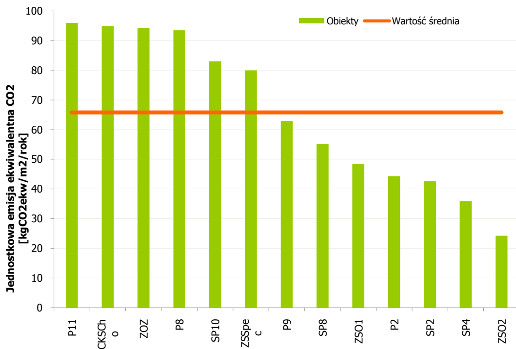
Rysunek 8-19 Porównanie jednostkowej emisji ekwiwalentnej CO 2 związanej z wytwarzaniem ciepła sieciowego dla poszczególnych obiektów
