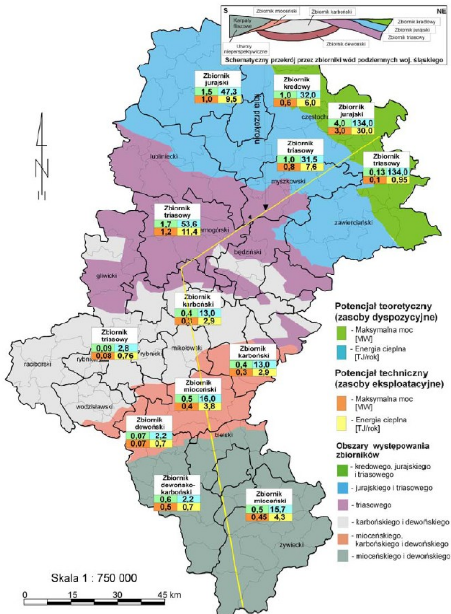
Rysunek 5-7 Zasoby energii geotermalnej na terenie województwa śląskiego
